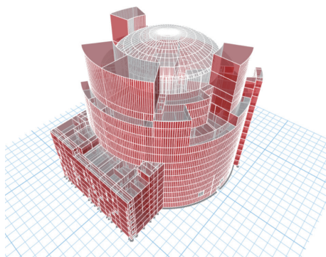
图 1 核岛厂房整体有限元模型 Fig. 1 Finite element model of nuclear island plant
